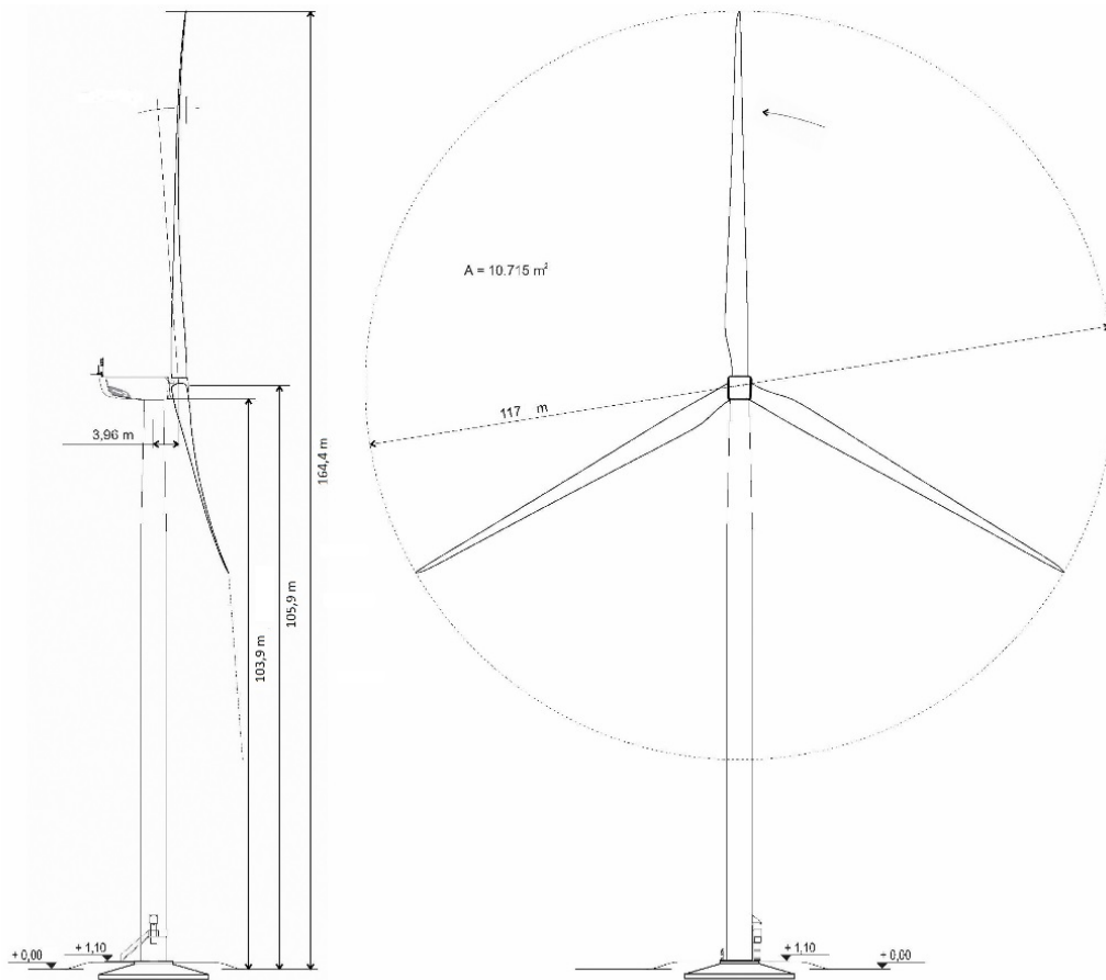
Figure 4 : Plans en coupe de l'éolienne N117 – 3,6MW – 164 m
